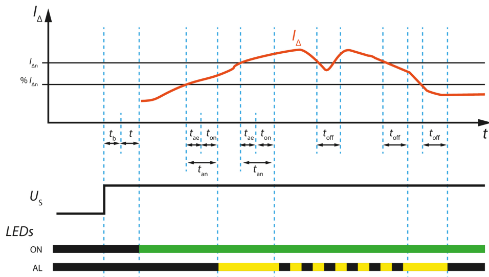
Abbildung 2-1: Zeitdiagramm
