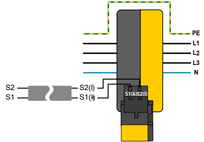
Messstromwandler „Typ A/Typ F“
